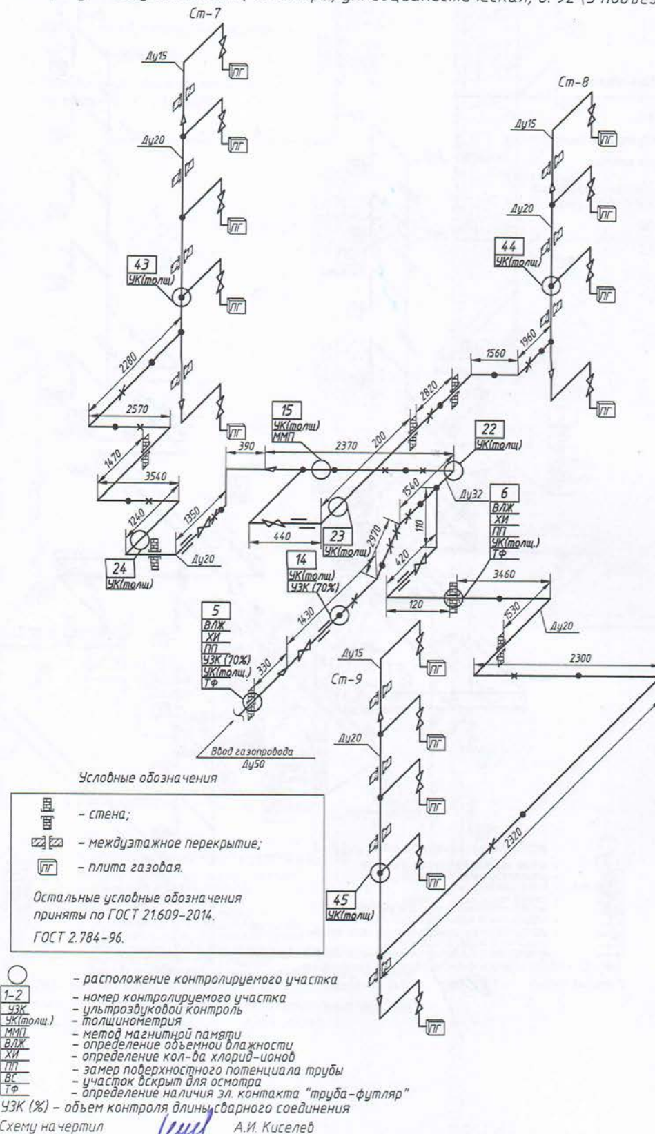
Схема неразрушающего контроля внутридомового газового оборудования по адресу: Республика Коми, г. Печора, ул. Социалистическая, д. 92 (3 подъезд)
