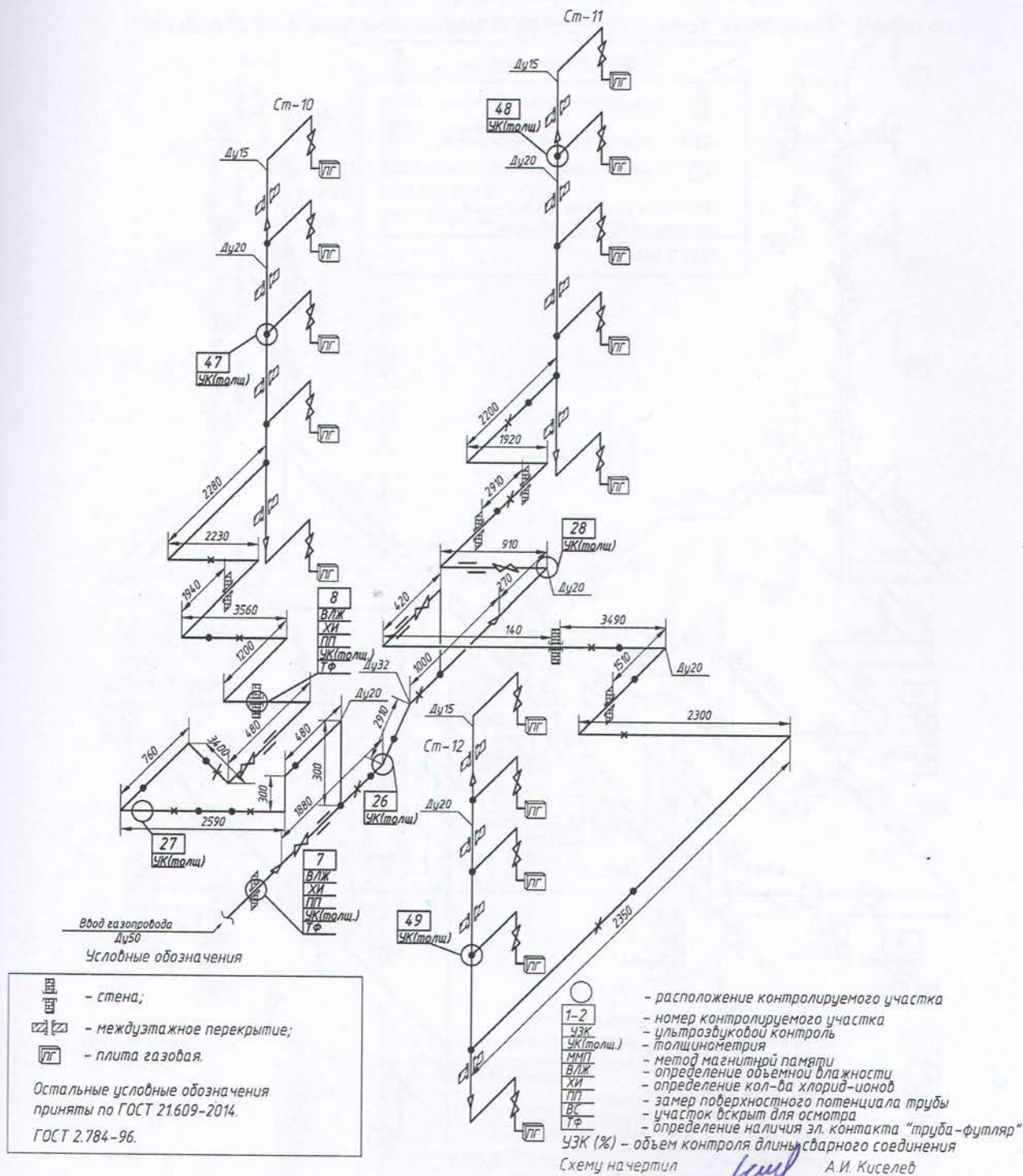
Схема неразрушающего контроля внутридомового газового оборудования по адресу: Республика Коми, г. Печора, ул. Социалистическая, д. 88 (4 подъезд)
